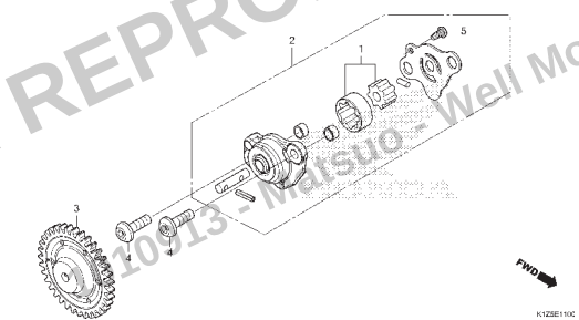
M-11 Bomba de Óleo
