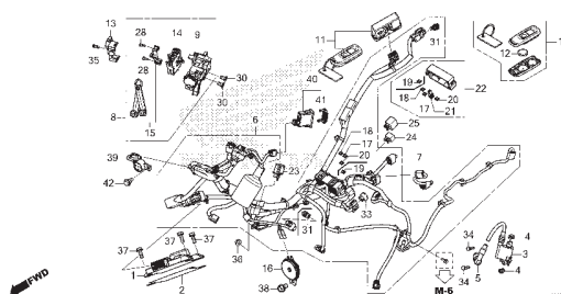
C-41.1 Fiação Principal • Chave FOB (2)
