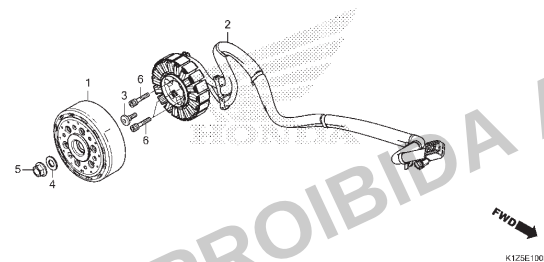
M-10 Motor de Partida A.C.G.
