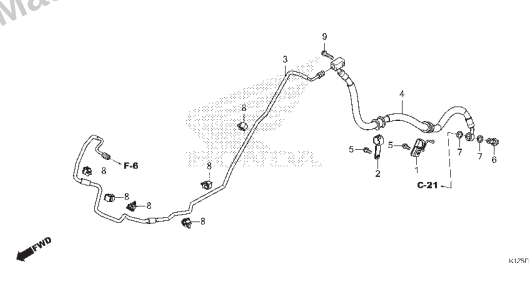
C-7.10 Tubo de Freio Traseiro
