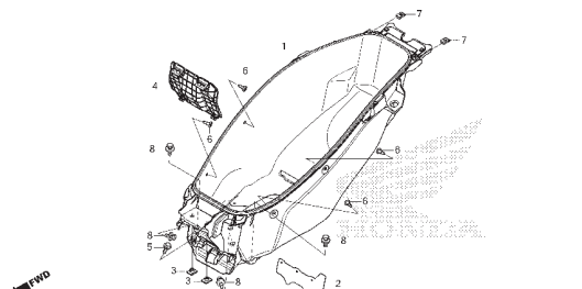
C-16 Compartimento de Bagagem
