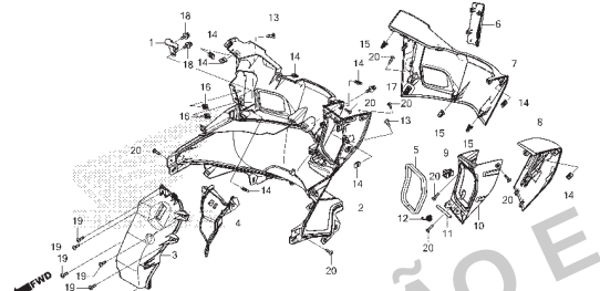
C-15 Tapa da Carcaça
